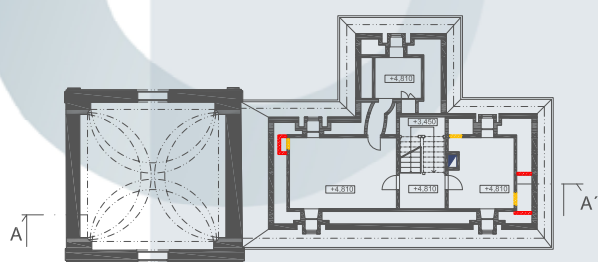
pôdorys 2.N.P. 1:150
