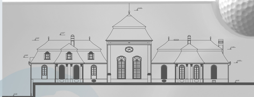
pohľad severo-východný 1:150
