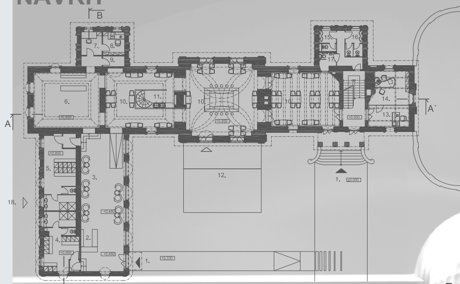
pôdorys 1.N.P. 1:150
