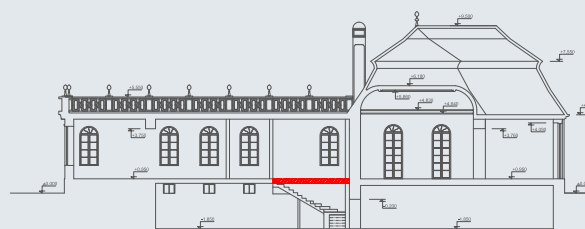
REZ B-B' 1:150
