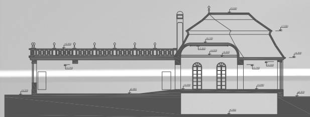
rez B-B' 1:150
