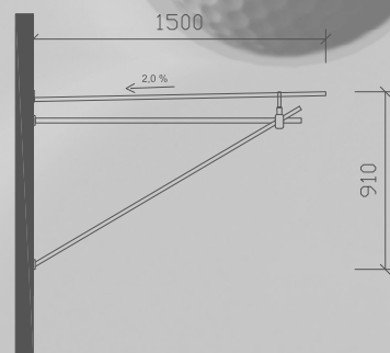
detail prestrešenia nového vstupu 1:10
