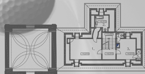
pôdorys 2.N.P. 1:150
